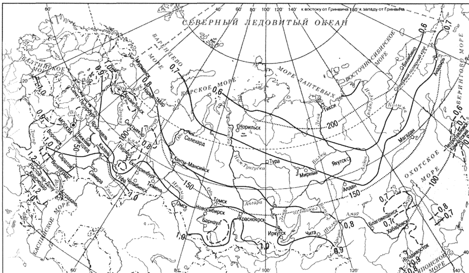
Рисунок 1— Климатические коэффициенты для определения величины нагрузки на иловые площадки (сплошные и пунктирные линии) и продолжительности периода намораживания на иловых площадках, дни (точечные линии)
